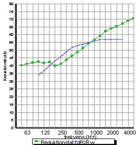
Fig. 2 Beräknat reduktionstal för en massiv och homogen betongplatta med tjockleken 138 mm som representerar det lägsta reduktionstalet som kan erhållas för direkttransmission genom skärmaterialet. Det visade reduktionstalet är R'_w + C_{tr} = 53 + (-4) \text{ dB} = 49 \text{ dB} . Sannolikt är reduktionstalet för Z-Bloc-skärmen ytterligare bättre än det som här redovisas.
